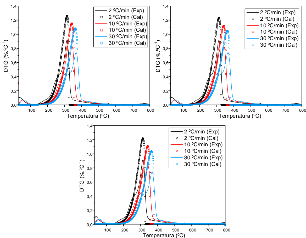
Figura 34. Comparação das curvas de DTG experimental e calculada para os métodos de (□) Friedman (○) FWO (Δ) KAS nas razões de aquecimento de 2, 10 e 30 °C.min -1
