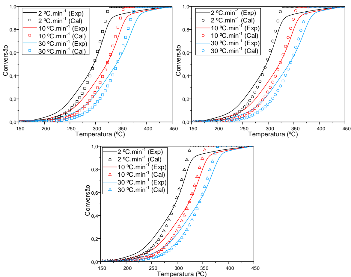
Figura 32. Comparação das curvas de conversão experimental e simuladas para os métodos de ( \square ) Friedman ( \circ ) FWO ( \Delta ) KAS nas razões de aquecimento de 2, 10 e 30 ^{\circ}\text{C}\cdot\text{min}^{-1}
